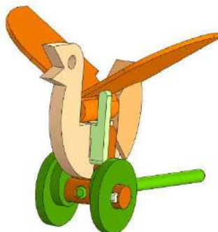
Рис.2 – Модель игрушки «Птица» с кулачковым механизмом
